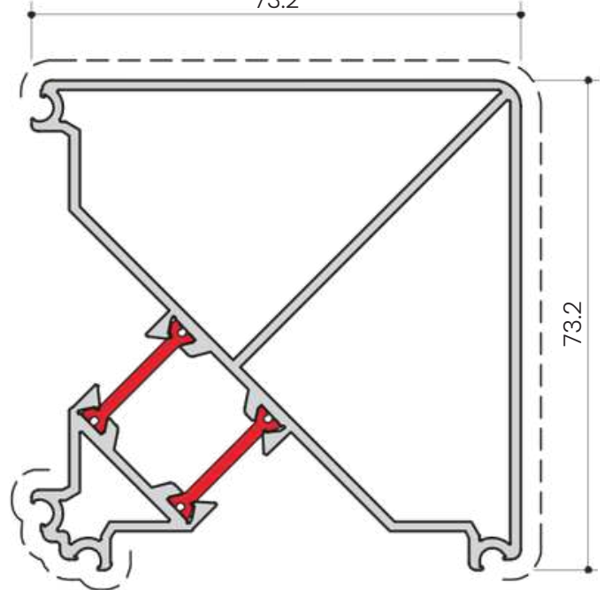
6754 POTEAU DE LIAISON A 90 73.2
