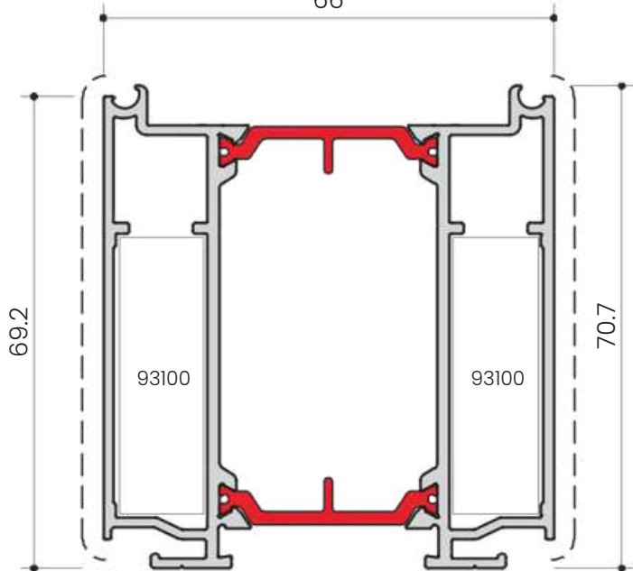
U99602 REHAUSSE 65 MM 66
