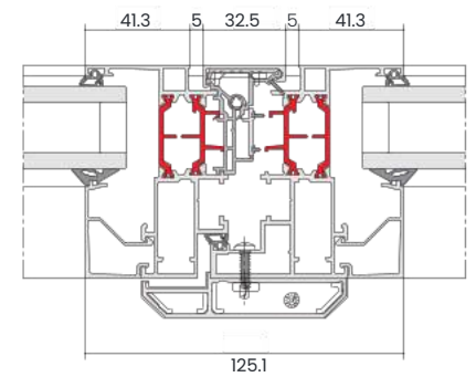
» 67FR MONTANT CENTRAL OUVRANT VISIBLE F22
