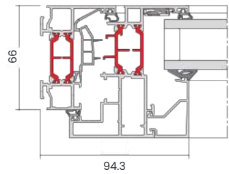
» 67FR MONTANT LATÉRAL OUVRANT VISIBLE F22
