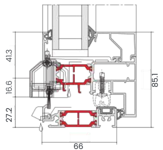
» 67FR TRAVERSE BASSE OUVRANT VISIBLE SEUIL PMR F37
