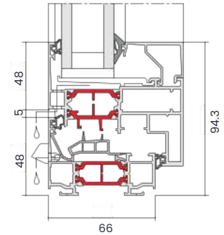
» 67FR TRAVERSE BASSE OUVRANT VISIBLE F22
