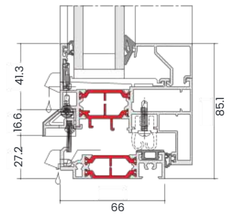
» 67FR TRAVERSE BASSE OUVRANT VISIBLE SEUIL PMR F22
